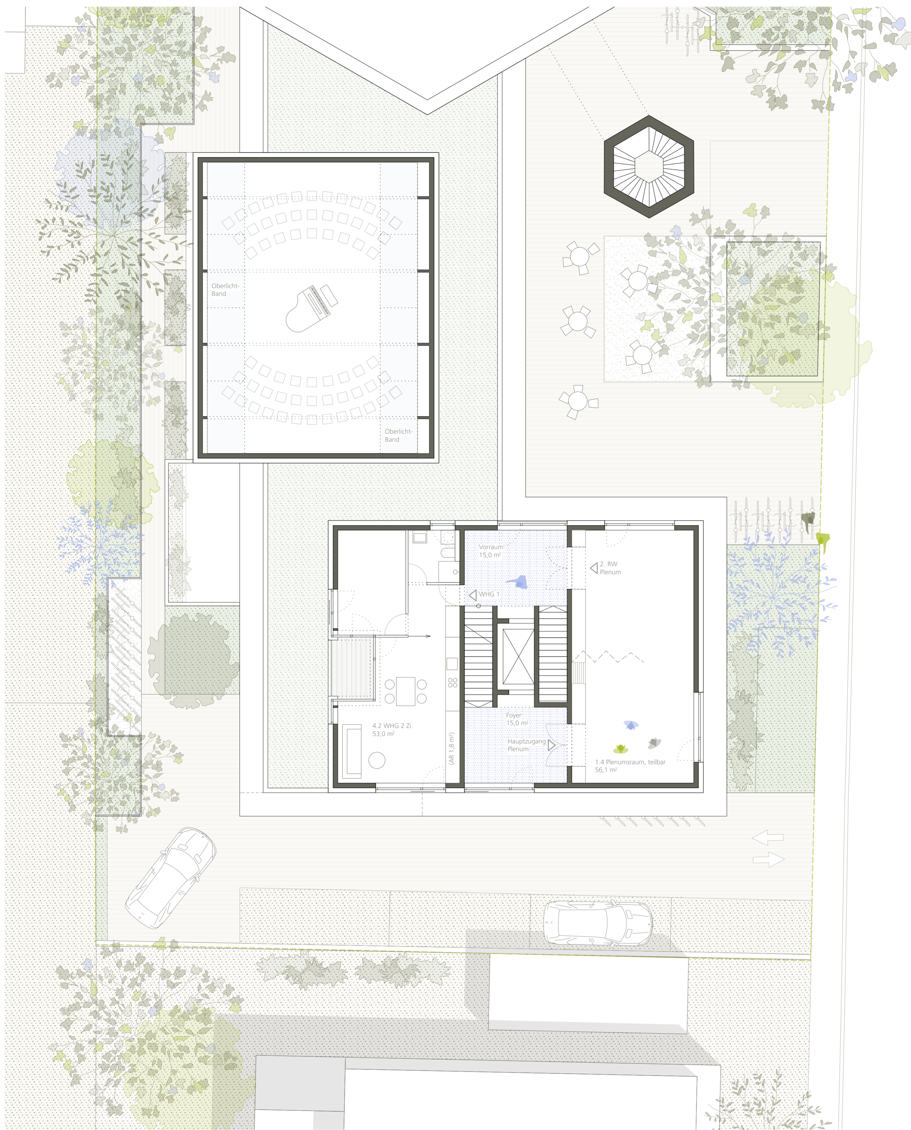
Grundriss Obergeschoss 1:100
