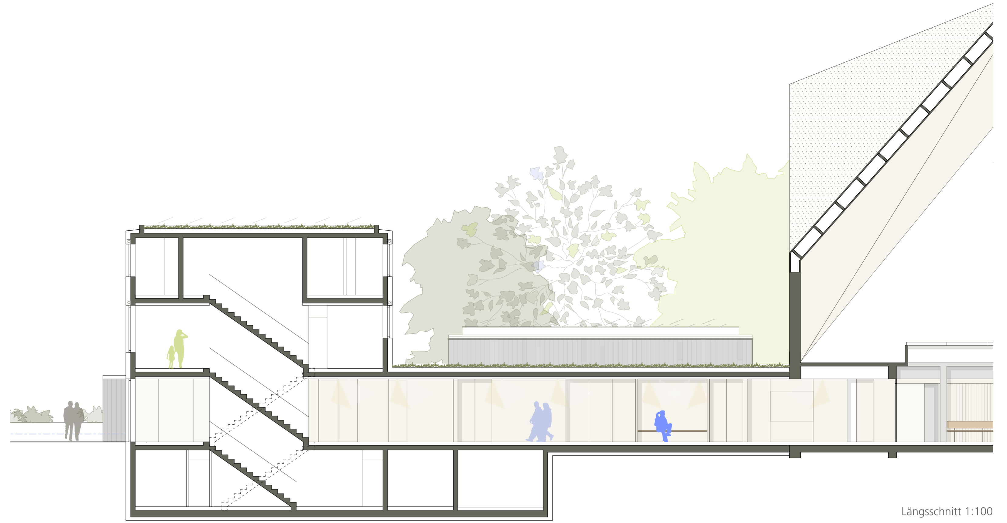
Längsschnitt 1:100
