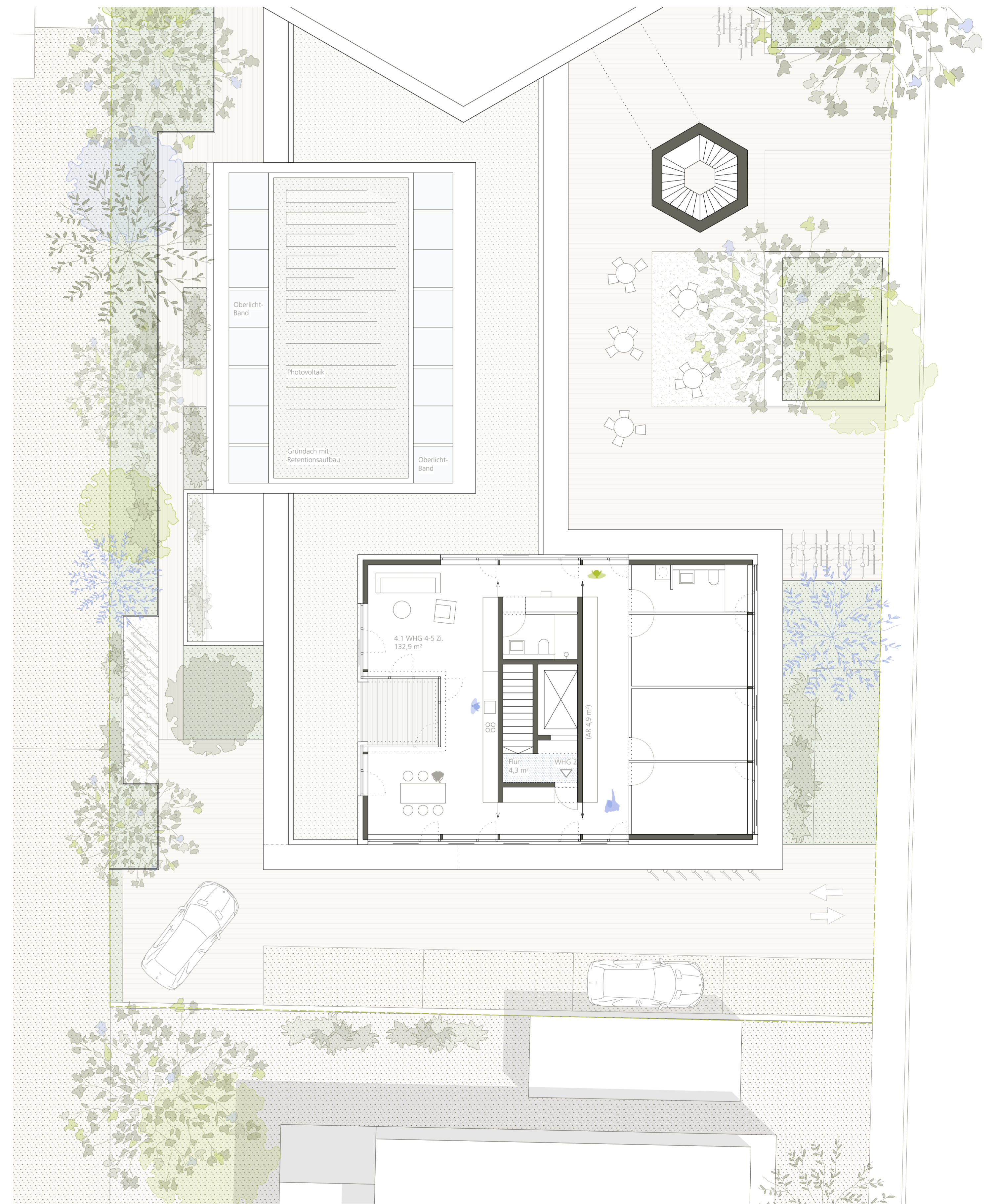
Grundriss Dachgeschoss 1:100
